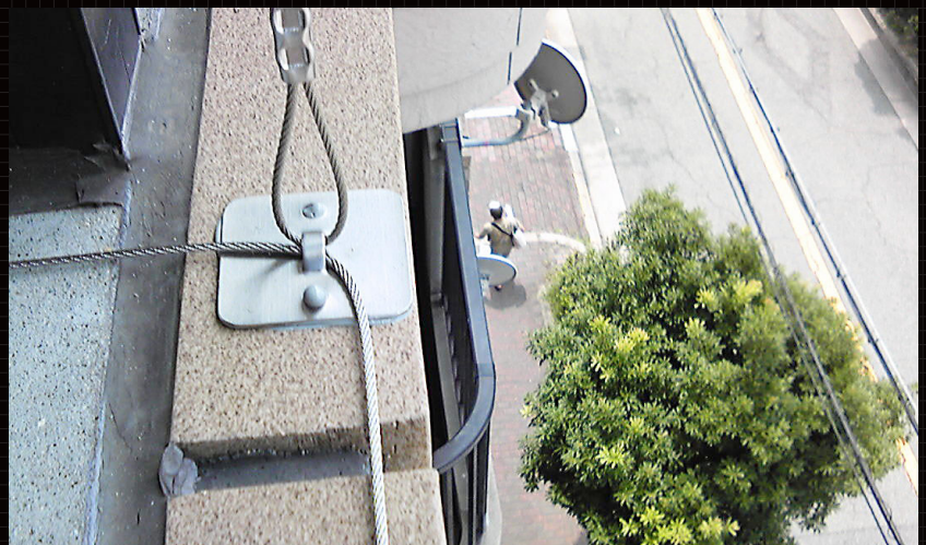
SUSプレート[SUS ワイヤーφ2.0+ ワイヤー固定具(AL)]
