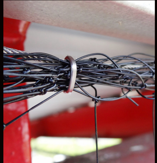
ホグリング [トリカットネット +SUS ワイヤーφ2.0]
